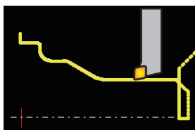
仕上げ加工
