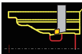
等高線荒取り加工
